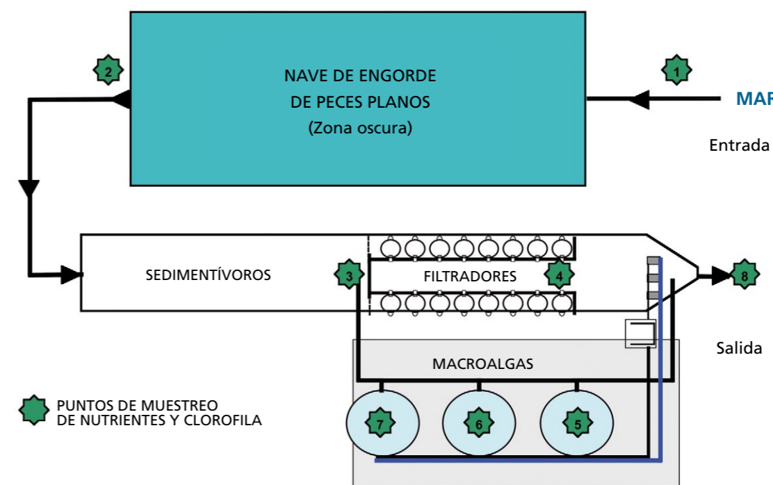
En el esquema se pueden ver los puntos de muestreo de nutrientes y de clorofila en la entrada del agua (1), después de pasar por los peces (zona oscura) (2), antes y después de pasar por los bivalvos (3 y 4), en el cultivo de algas (5, 6 y 7) y en la salida de la instalación (8).
